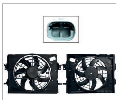
MOTOVENTILADOR COMPLETO C/S AIRE C/TOLVA S/RES 2PIN (KICKS 17-24)
