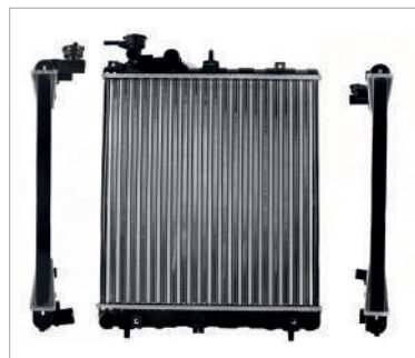
RADIADOR AGUA S/AIRE STD 400*430*22MM T/MECANICO
