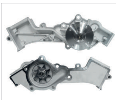
BOMBA AGUA (PATHFINDER 3.3L/X-TERRA 3.3L)
