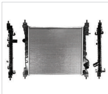
RADIADOR AGUA C/S AIRE STD 450*390*16MM T/SOLDADO (BEAT 1.2L 18-21)
