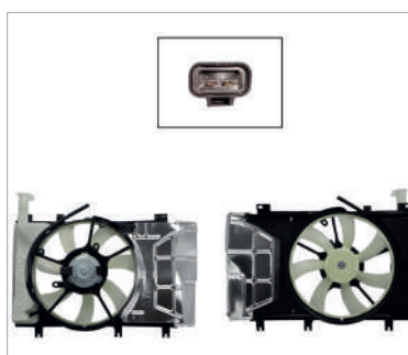
MOTOVENTILADOR COMPLETO C/S AIRE C/TOLVA C/DEPOSITO S/RES 2PIN
