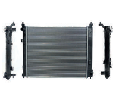
RADIADOR AGUA C/S AIRE STD 520*430*20MM (V-DRIVE/MARCH/NOTE/MICRA) T/SOLDADO
