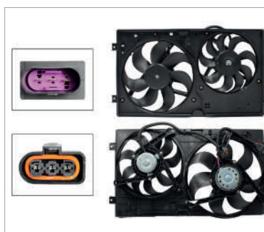
MOTOVENTILADOR COMPLETO C/AIRE C/TOLVA S/RES 3PIN (2ASPAS)
