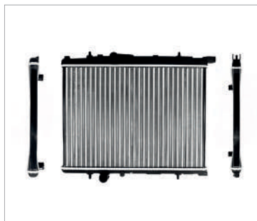
RADIADOR AGUA C/S AIRE STD 550*400*22MM T/MECANICO
