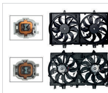
MOTOVENTILADOR COMPLETO C/S AIRE C/TOLVA S/RES PIN (2ASPAS)
