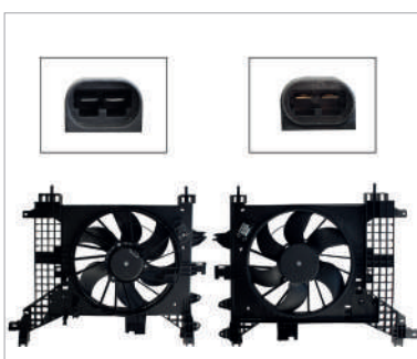
MOTOVENTILADOR COMPLETO C/AIRE C/TOLVA C/RES 2PIN
