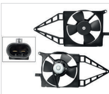
MOTOVENTILADOR COMPLETO S/AIRE C/TOLVA S/RES 2PIN (C-2/C-3)
