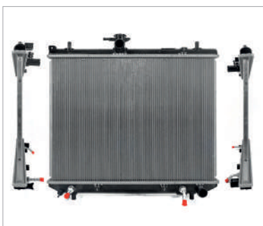
RADIADOR AGUA C/S AIRE AUT 570*450*16MM T/SOLDADO
