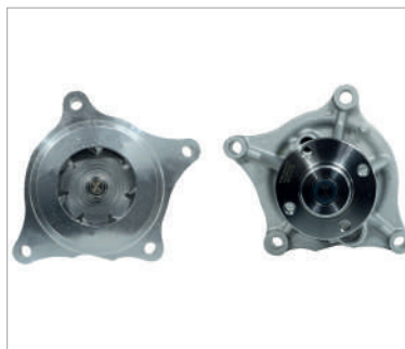
BOMBA AGUA (F-250 F-350 6.2L SUPER DUTY/E-350 6.2L SUPER DUTY)
