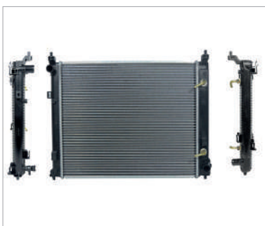
RADIADOR AGUA C/S AIRE AUT 520*430*20MM (V-DRIVE/MARCH/NOTE/MICRA) T/SOLDADO
