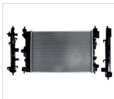
RADIADOR AGUA C/S AIRE STD 580*390*16MM T/SOLDADO
