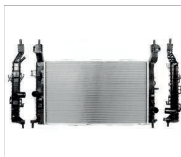
RADIADOR AGUA C/S AIRE STD 610*370*26MM T/SOLDADO
