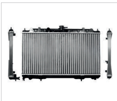
RADIADOR AGUA C/S AIRE STD 710*380*26MM (SCALA 1.6L 10-13) T/MECANICO
