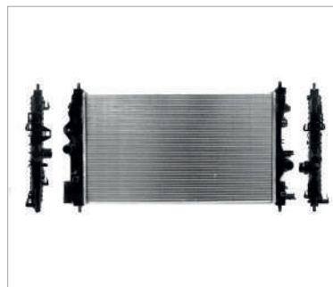
RADIADOR AGUA C/S AIRE STD 700*410*26MM T/SOLDADO
