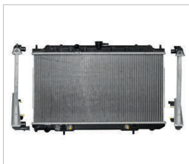
RADIADOR AGUA C/S AIRE AUT 710*380*16MM (SCALA 1.6L 10-13) T/ SOLDADO
