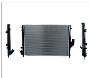
RADIADOR AGUA C/S AIRE STD/AUT 600*410*26MM (SANDERO-STEPWAY 15-16) T/SOLDADO
