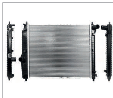
RADIADOR AGUA S/AIRE STD 500*440*16MM (PT G3 06-09) T/SOLDADO
