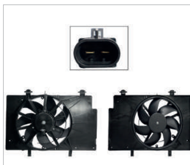
MOTOVENTILADOR COMPLETO S/AIRE C/TOLVA S/RES 2PIN (FIESTA 11-19/ECOSPORT 13-17)
