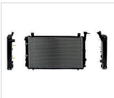
RADIADOR AGUA C/S AIRE STD/AUT 610*350*16MM 8VAL T/SOLDADO
