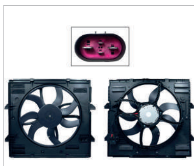
MOTOVENTILADOR COMPLETO C/AIRE C/TOLVA C/RES 4PIN (MOTOR DC)
